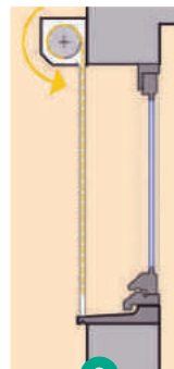
3 Posé devant linteau (Dispo 3)
