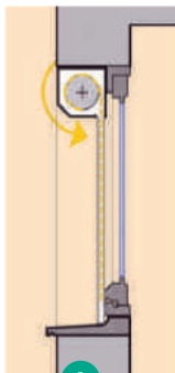
1 Posé sous linteau en enroulement extérieur (Dispo 1)
